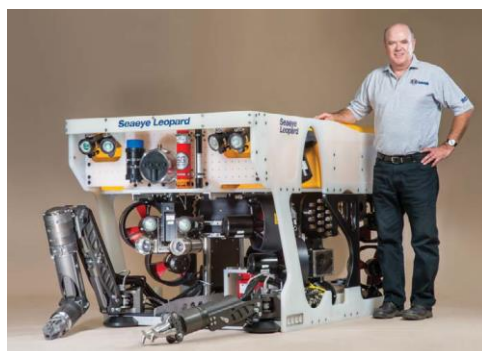
LEOPARD 2000/3000m 大水深オプション可能
